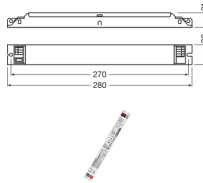
Spesifikasjoner Osram LED Driver OPTOTRONIC 55/220-240/1A0 CS L G2
